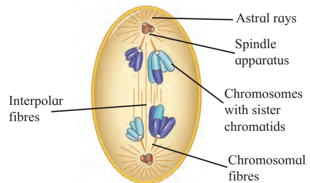
Fig. 7.9 Anaphase-I
